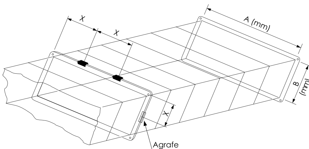
(Fig.d) Agrafe boulonnée pour cadre M et HM
